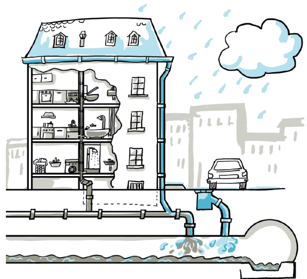
Abb. 2: Mischsystem
