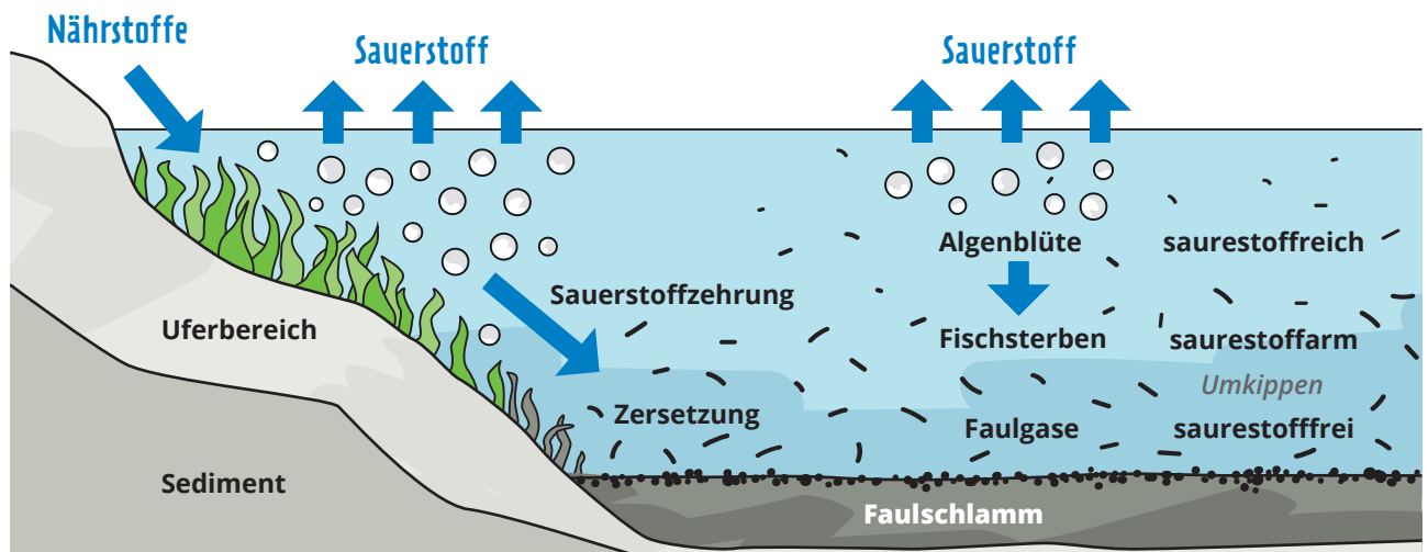
Abb. 3: Prozess der Eutrophierung
